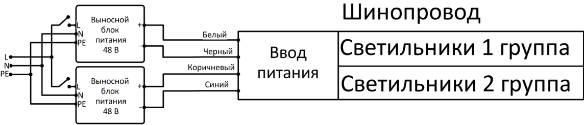
Пример схемы с двумя выносными блоками питания
